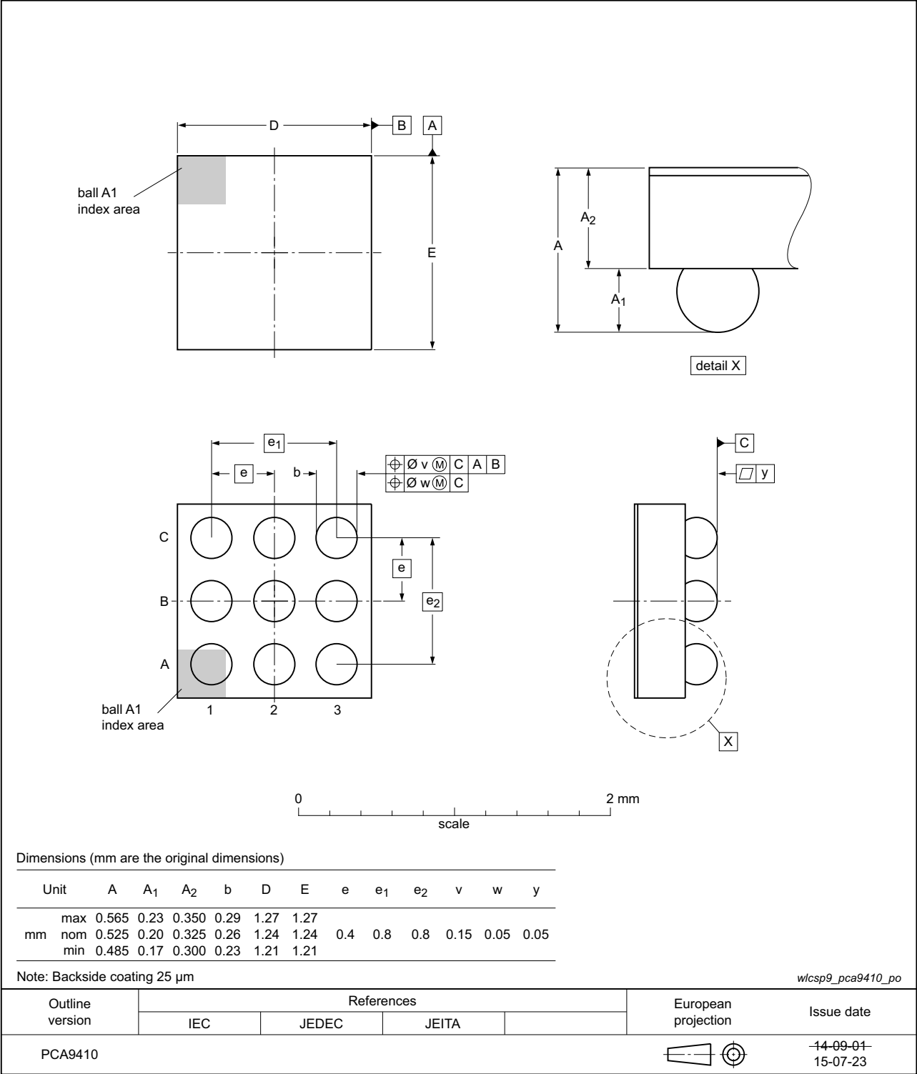
Fig 20. Package outline WLCSP9
