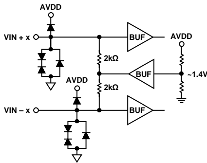
Figure 27. Analog Inputs
