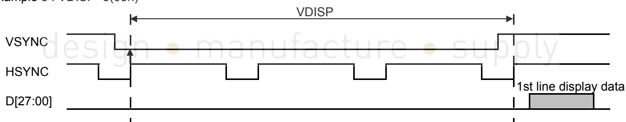
Example 4 : VDISP=0(00h)
