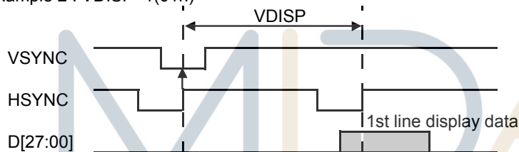
Example 2 : VDISP=1(01h)
