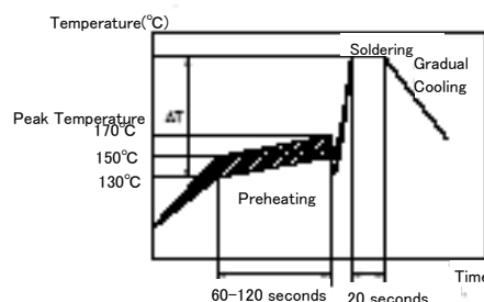
Vapor Reflow
