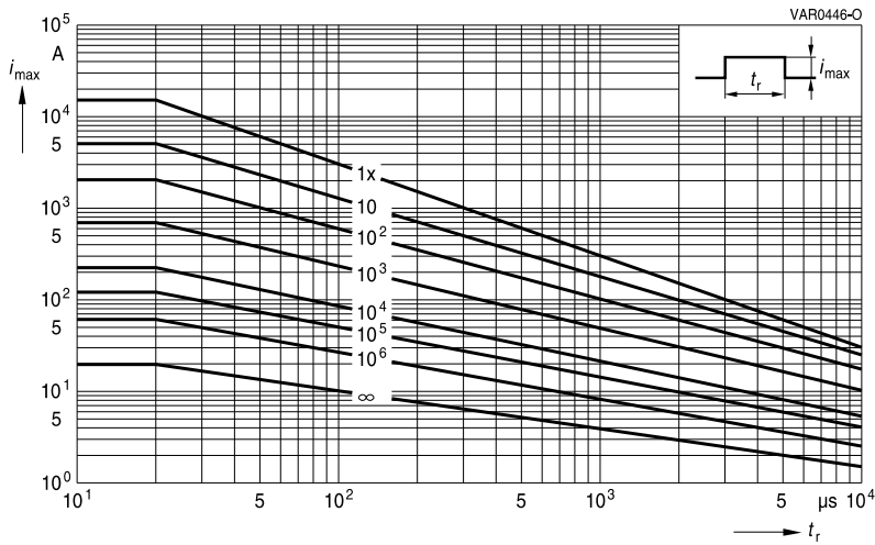
SIOV-Q20K130 ... K320
