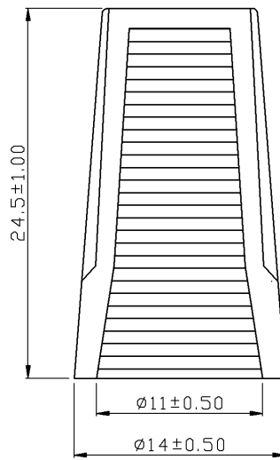
Dimensions : Millimetres
