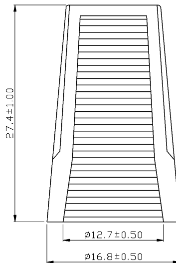
Dimensions : Millimetres
