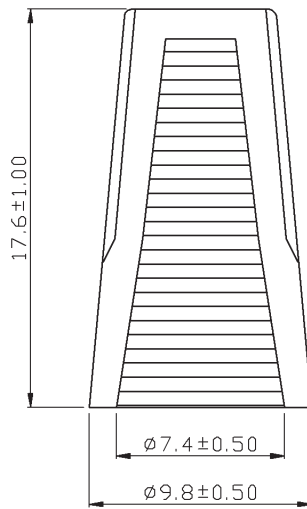
Dimensions : Millimetres
