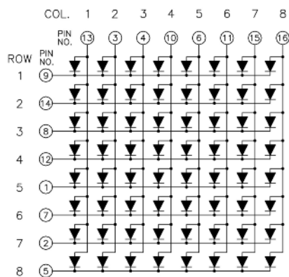
Column Anode
