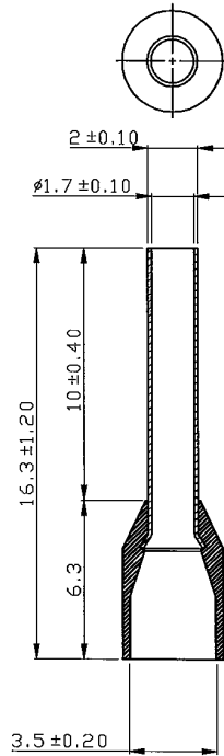
Dimensions : Millimetres
