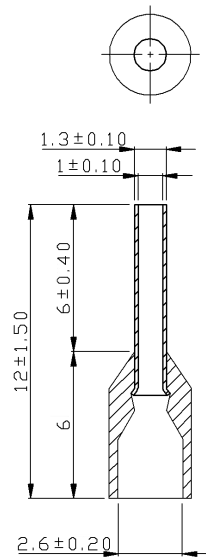
Dimensions : Millimetres
