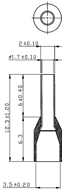
Dimensions : Millimetres
