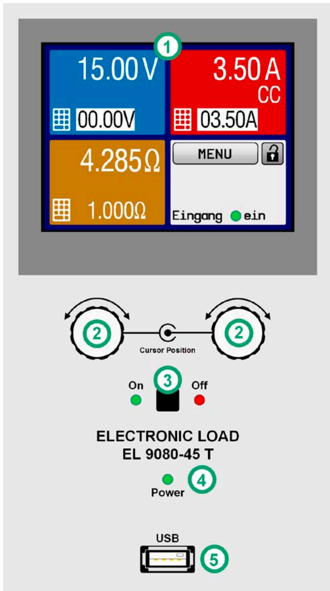
Bild 5- Bedienfeld
