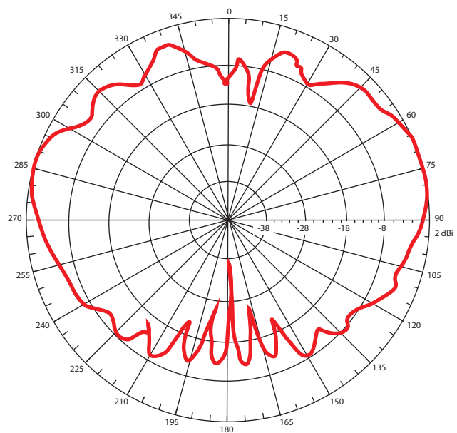
E-PLANE
