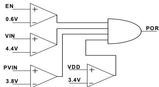
FIGURE 29. POR CIRCUIT
