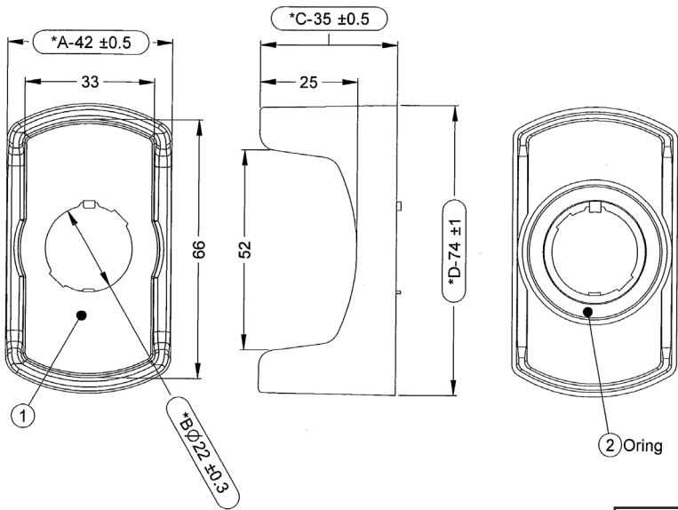
Dimensions : Millimetres
