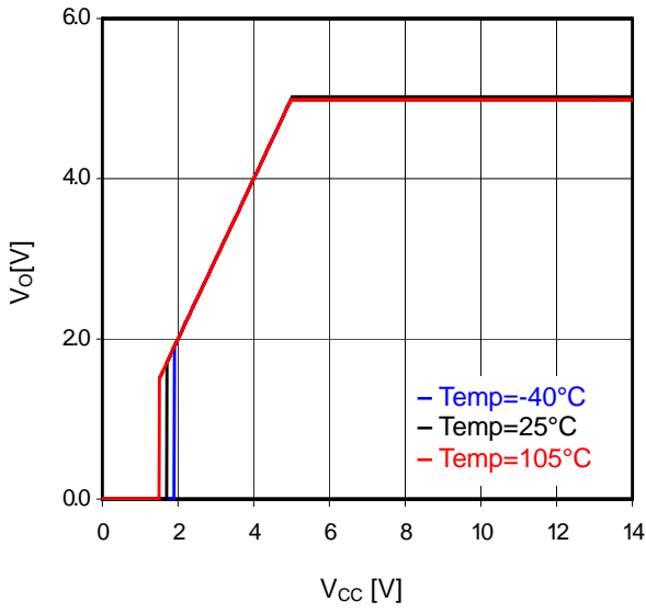
Fig. 27 V_{CC}-V_O ( I_O=0mA )
