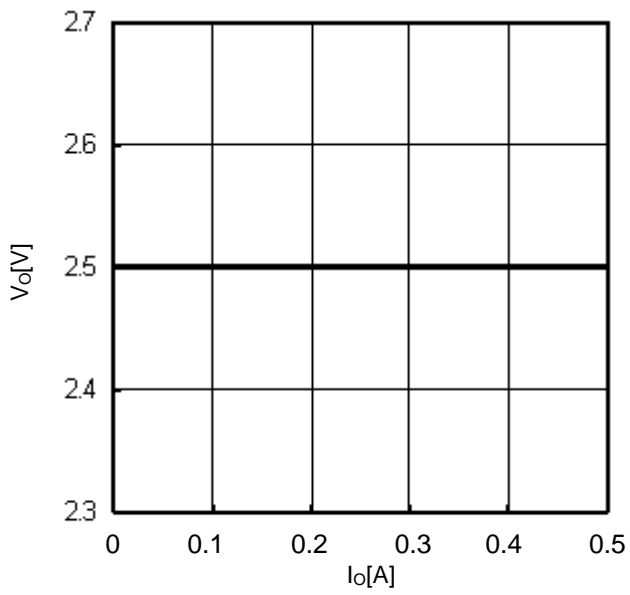
Fig.13 I_O - V_O
