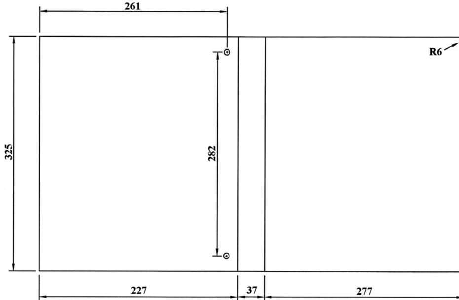
Dimensions : Millimetres
