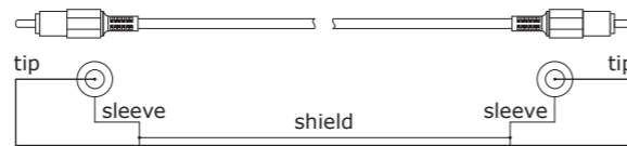
Fig. 3.5: RCA cable
