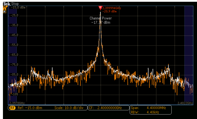
Automatische Kanalleistungsmessung
