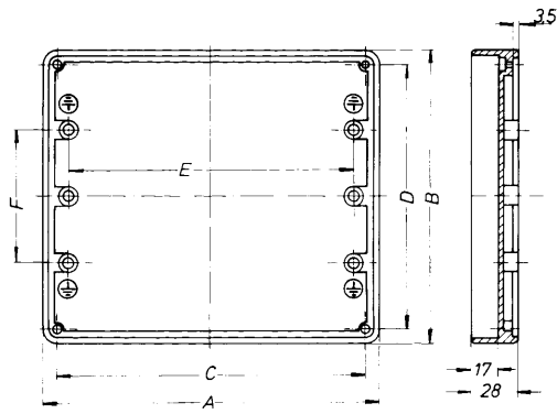
Aluminium cast bezel lid
