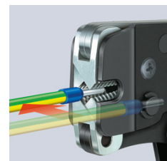
97 53 08: Einführen von Aderendhülsen parallel von der Seite bis 2,5 mm 2 z. B. unter beengten Platzverhältnissen
