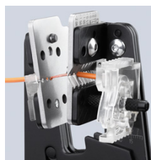
Exakt avisolering genom exakta knivprofiler
