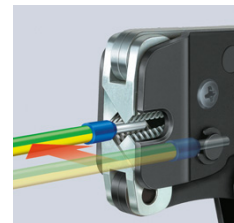
97 53 08 innføring av lederendehylser parallelt fra siden inntil 2,5 mm 2 f.eks under trange plassforhold
