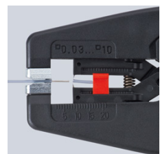
Descarnar com precisão de 0,03 até 10 mm 2 sem reajuste
