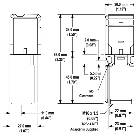
Model SI-QS-SSU Flexible Actuator
