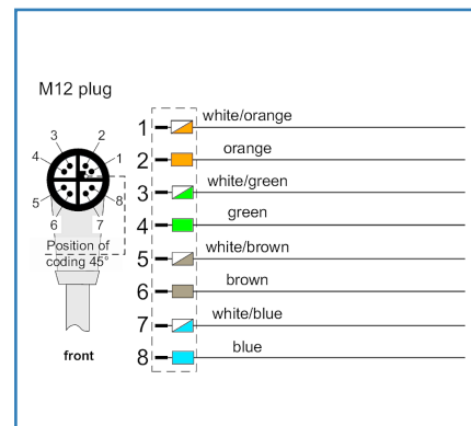
Anschlussbild 142M2XA0xxx
