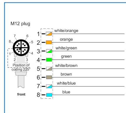
Anschlussbild 142M2XC0xxx
