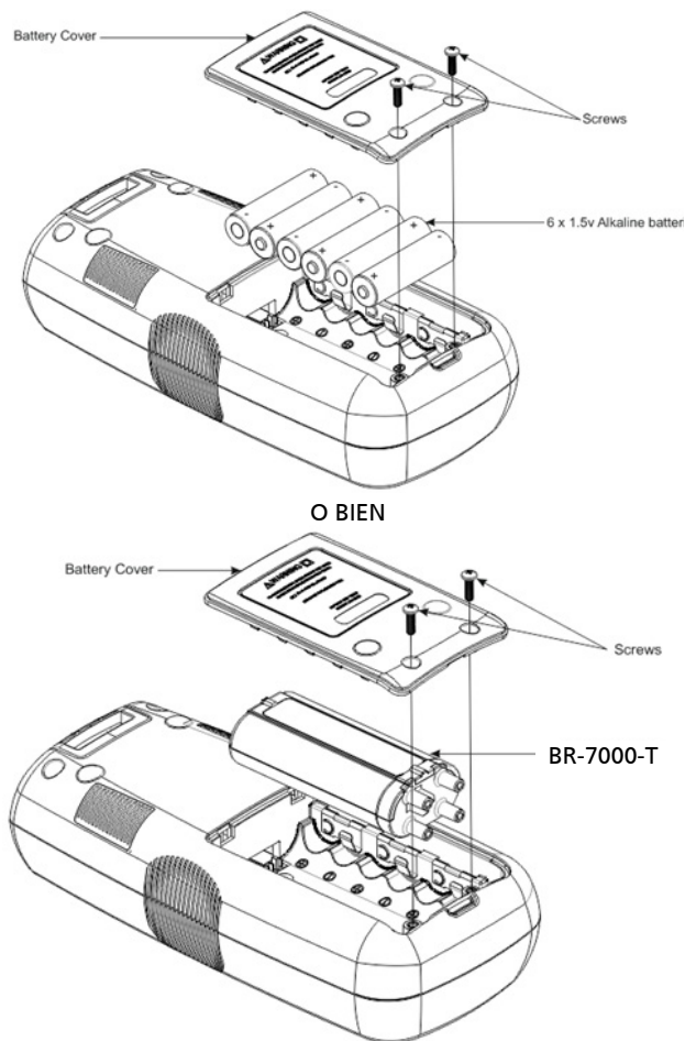
Figura 5.1: Cambio de las pilas del transmisor
