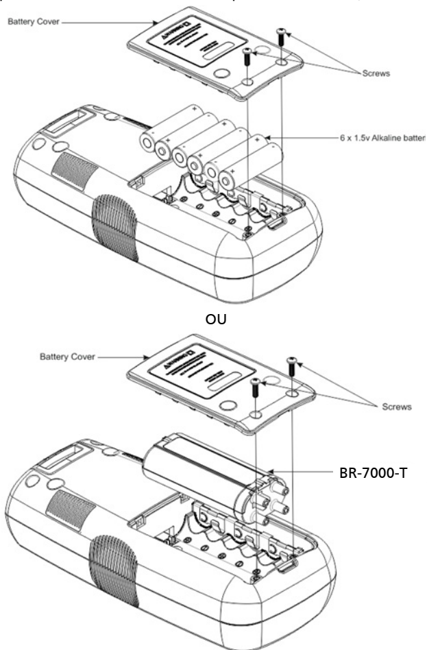
Figure 5.1 : Changer les piles du transmetteur
