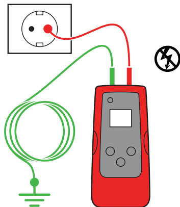
Obr. 3.3a Správné připojení s odděleným uzemněním
