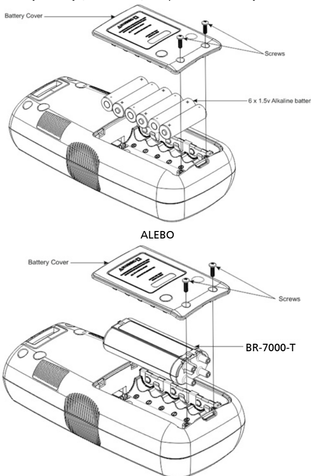
Obrázok č. 5.1: Výmena batérií vo vysieläči
