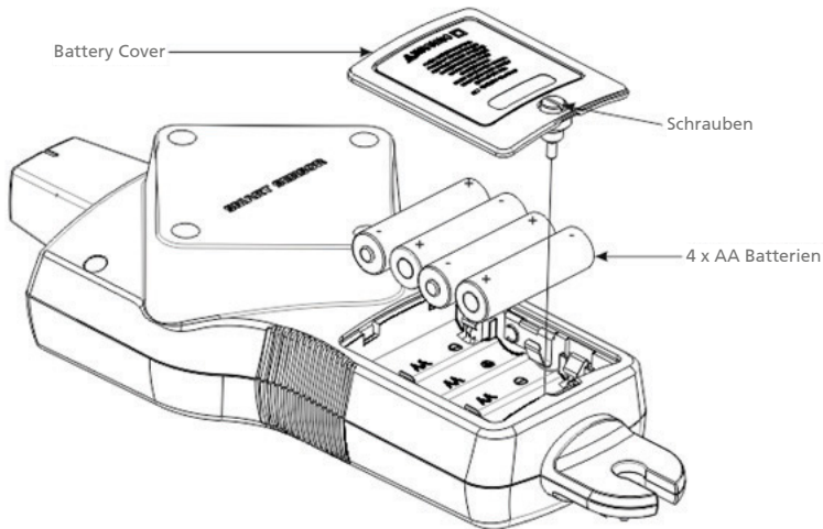
Abbildung 5.2: Empfängerbatterien wechseln
