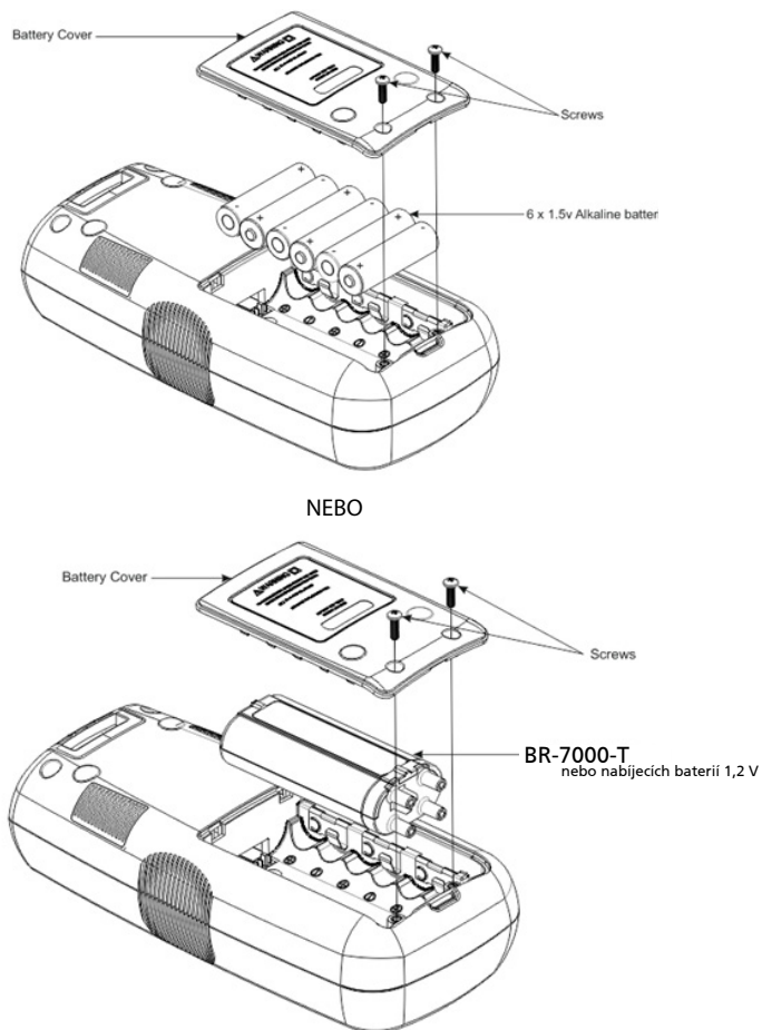
Obr. 5.1: Výměna akumulátoru/baterií vysílače
