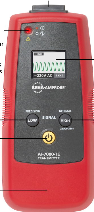
Figure 2 : Vue d'ensemble du transmetteur AT-7000-TE
