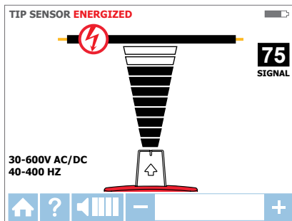
Приемник, показывающий сигнал, обнаруженный в режиме «ШТЫРЕВОЙ ДАТЧИК под напряжением».
