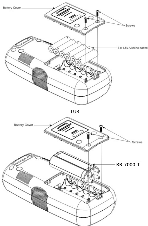
Rysunek 5.1: Zmiana baterii nadajnika
