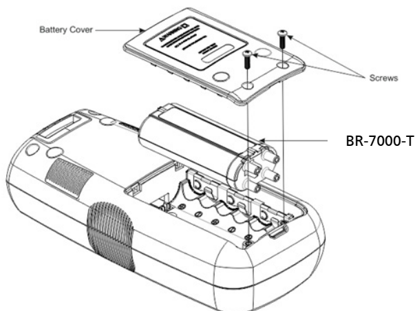
Рис. 5.1. Замена батареи передатчика
