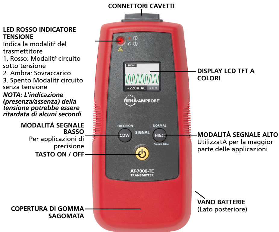
Figura 2: Descrizione del trasmettitore AT-7000-TE
