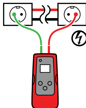
Figure 3.2a Connexion appropriée avec mise à terre séparée
