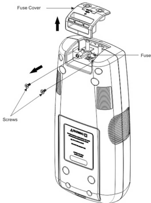
Kuva 5.4: Lähettimen sulakkeen vaihtaminen
