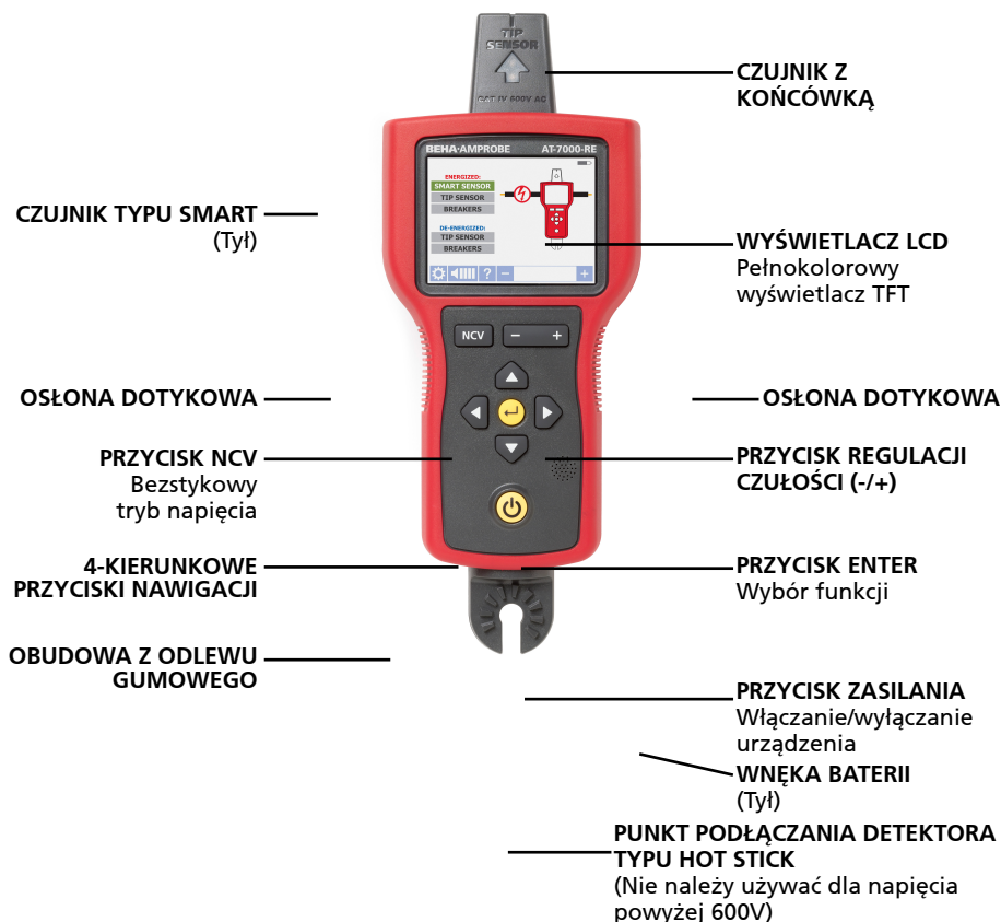
Rysunek 1: Przegląd odbiornika AT-7000-RE
