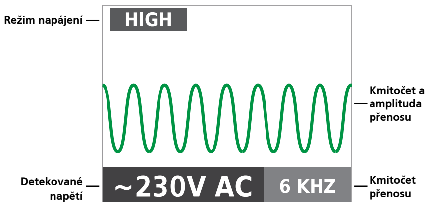
Obrázek 2a: Přehled LCD obrazovky vysílače AT-7000-TE
