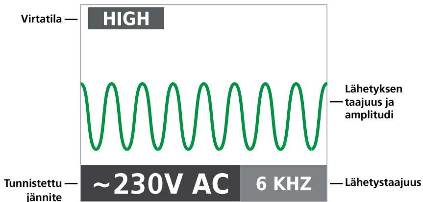
Kuva 2a: AT-7000-TE-lähettimen LCD-näytön yleiskatsaus
