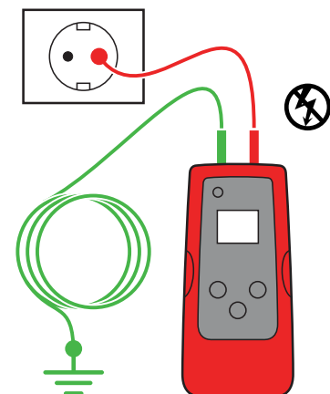
Figure 3.3a Connexion appropriée avec mise à terre séparée
