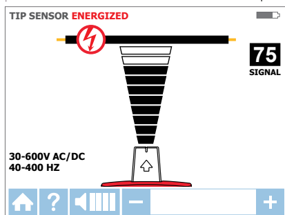
Figura 3.2e Ricevitore che mostra il segnale rilevato in modalit  SENSORE PUNTA sotto tensione
