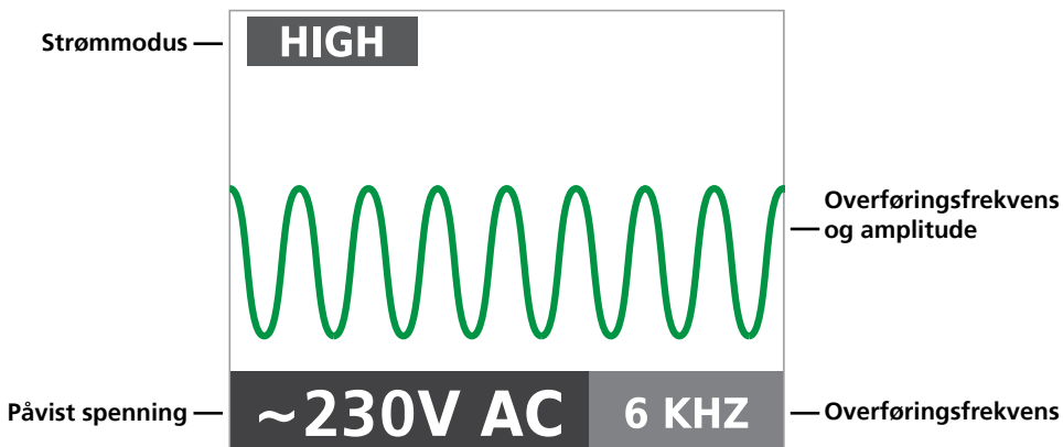
Figur 2a: Oversikt over LCD-skjermen på AT-7000-TE-sender
