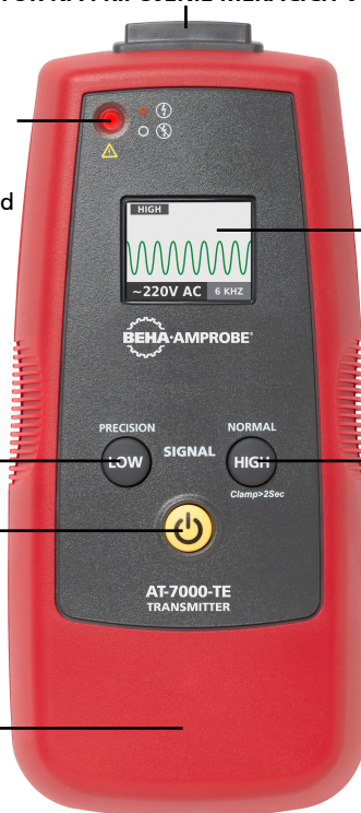
Obrázok č. 2: Prehľad vysielača AT-7000-TE
