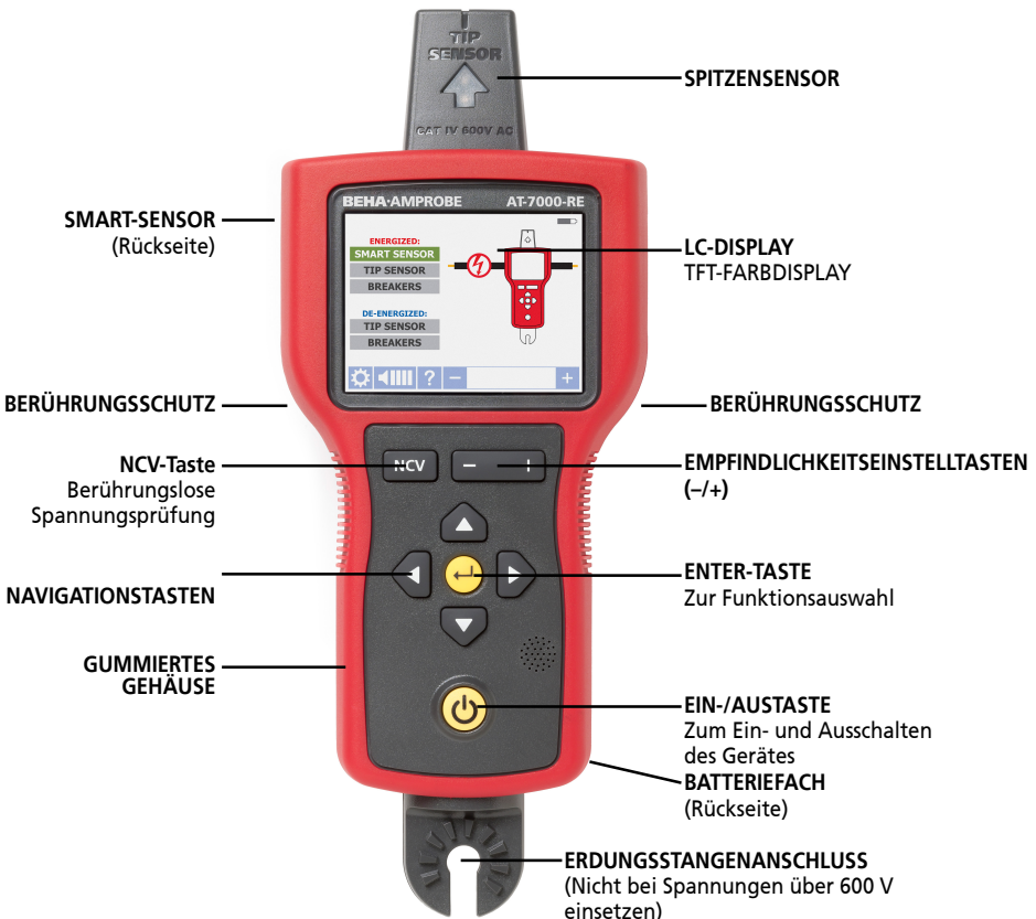
Abbildung 1: Empfänger AT-7000-RE – Überblick
