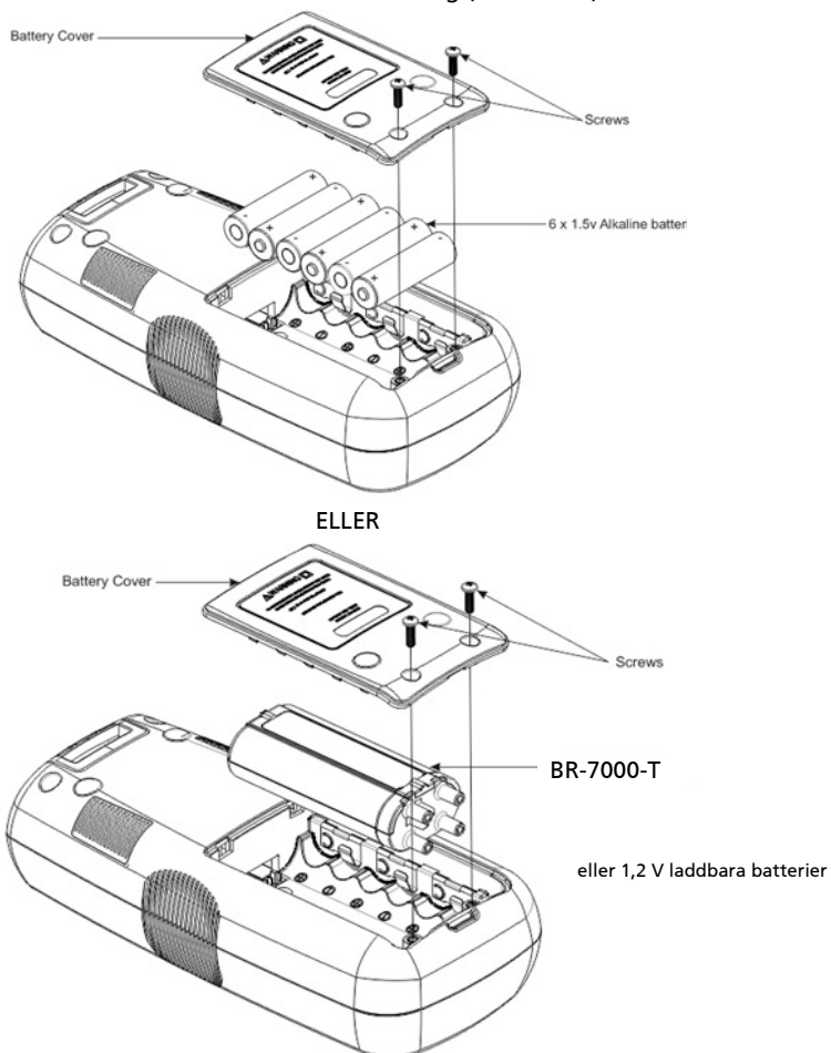
Figur 5.1: Byta sändarens batteri
