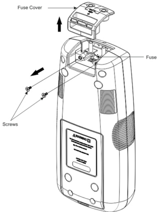
Afbeelding 5.4: De zekering van de zender vervangen
