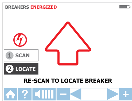
Afbeelding 3.4c ZOEKEN-modus – ontvanger die de stroomonderbreker/ zekering controleert
