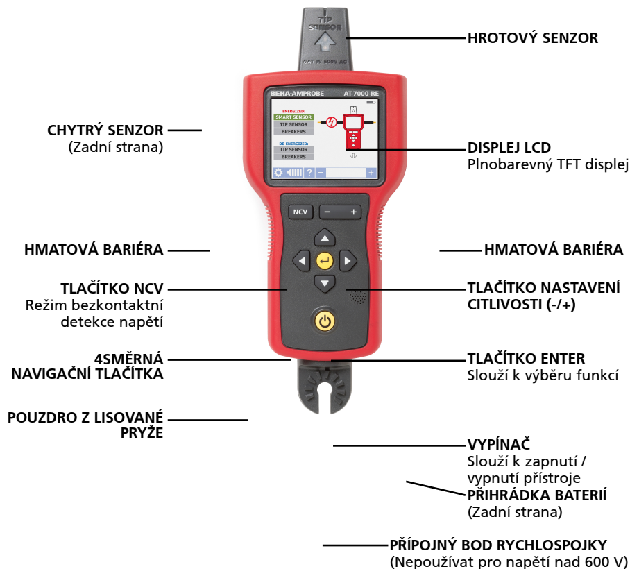
Obrázek 1: Přehled přijímače AT-7000-RE
