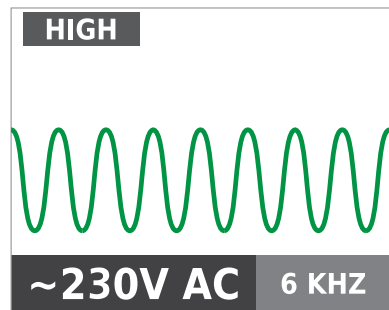
Obrázok č. 3.1b Displej vysielča zobrazuje signál v režime VYSOKÝ s frekvenciou 6 kHz pre obvod pod napätím
