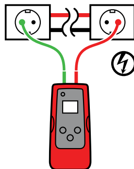
Rysunek 3.1a Prawidłowe podłączenie z oddzielnym uziemieniem
