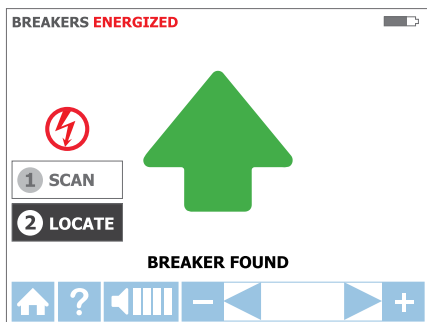
Afbeelding 3.4e ZOEKEN-modus – ontvanger die de stroomonderbreker heeft geïdentificeerd
