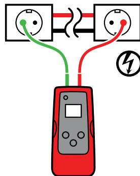
Rysunek 3.2a Prawidłowe podłączenie z oddzielnym uzziemieniem
