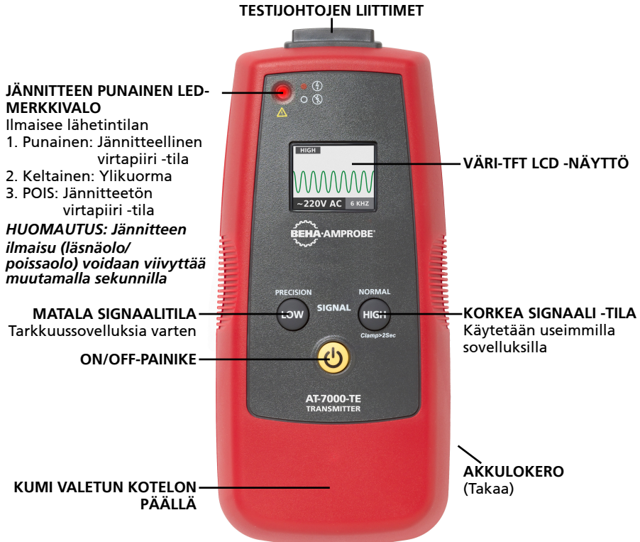
Kuva 2: AT-7000-TE-lähettimen yleiskatsaus
