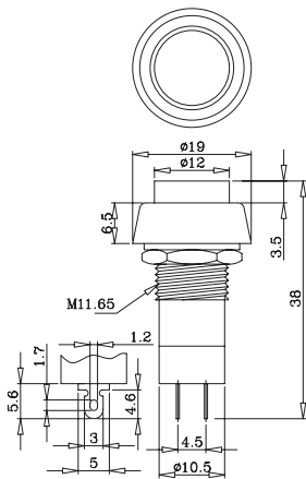
Dimensions : Millimetres
