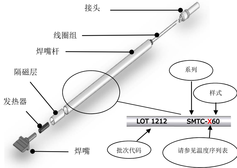
焊嘴结构与识别
