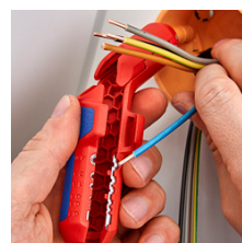
Afisolering af enkelte ledere
