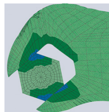
Tenaza llave: Presión superficial libre de juego, sin dañar los cantos
