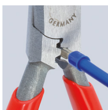
Sertissage de 0,5 à 2,5 mm 2
