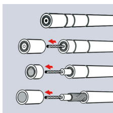
Dénudage en trois étapes d'un câble coaxial
