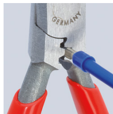
Crimpaggio da 0,5 a 2,5 mm 2
