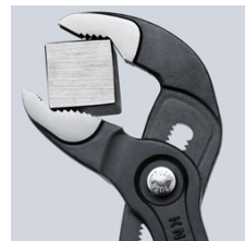
I denti contrari al senso di rotazione provocano un effetto autoserrante ed impediscono lo scivolamento sul pezzo.
