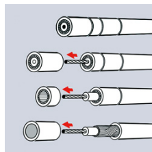
Tretrinns avisolering av en koax-kabel
