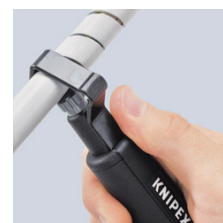
Csavarvonal menti vágás
