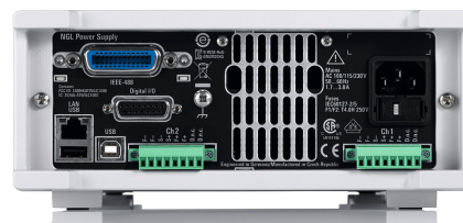
R&S®NGL202 Rückansicht
