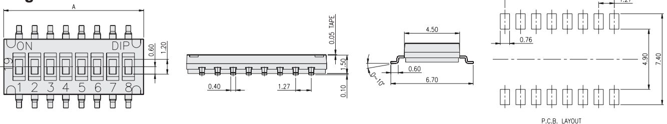
P.C.B. LAYOUT
