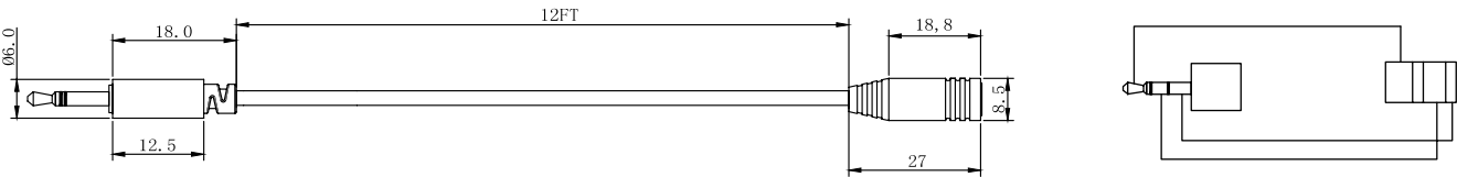
Dimensions : Millimetres
