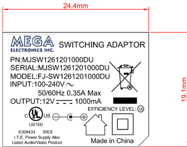
比例/Scale: 3:1
