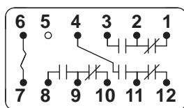
219XCX (3PDT)
