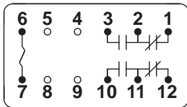
219XBX (DPDT)
