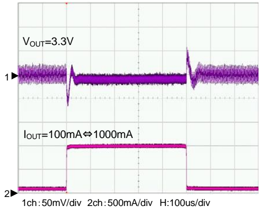
MYRGM330150B31RA ( V_{IN}=5V , I_{OUT}=100mA \leftrightarrow 1000mA )
