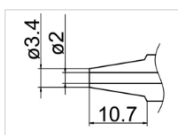
N3-20 Nozzle Size Φ2.0
