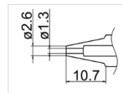
N3-13 Nozzle Size Φ1.3
