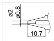
N3-08 Nozzle Size Φ0.8
