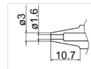
N3-16 Nozzle Size Φ1.6
