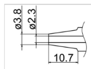
N3-23 Nozzle Size Φ2.3
