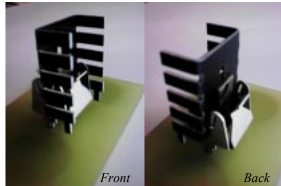
◆ 6030PB-CL07
