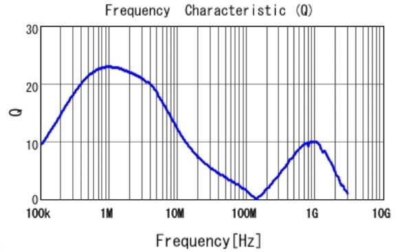
■ 1225AS-H-2R2M Q
