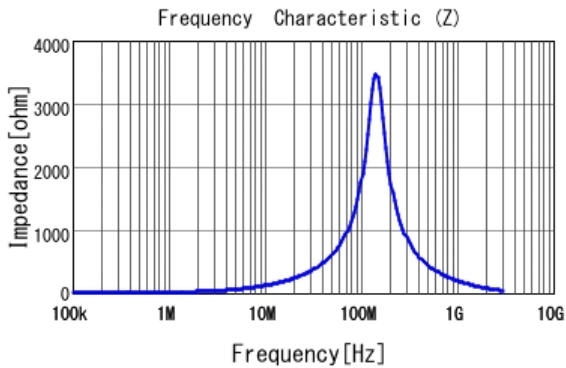
■ 1225AS-H-2R2M |Z|
