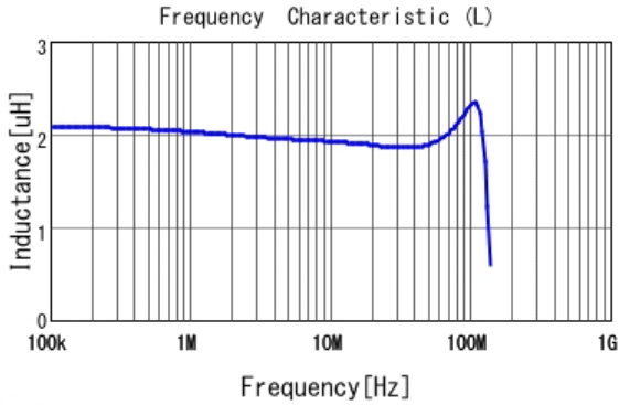
■ 1225AS-H-2R2M L
