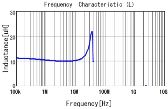
■ 1231AS-H-100M L
