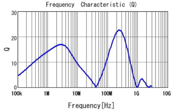
■ 1231AS-H-100M Q
