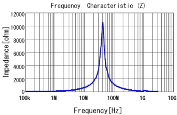
■ 1231AS-H-100M |Z|
